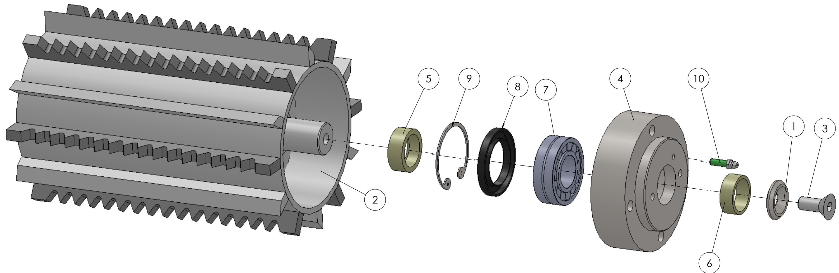
BOTTOM ROLLER
